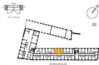
amm1104_StudentenwohnheimSteyr_Verkaufsplaene_Top06
